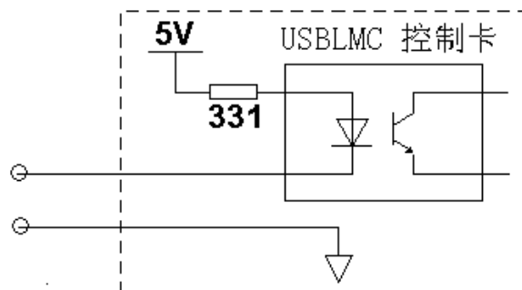
图 2-7 通用输入信号 (In4-8/XORG0/YORG0/Remark) 的接口电路示意图
