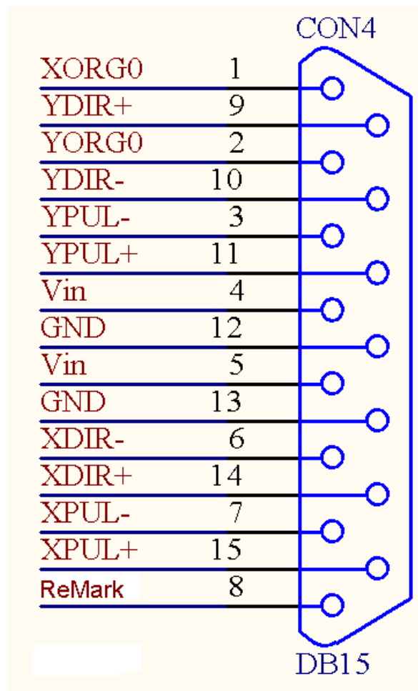
图 2-4 CON4 插座管脚定义示意图
