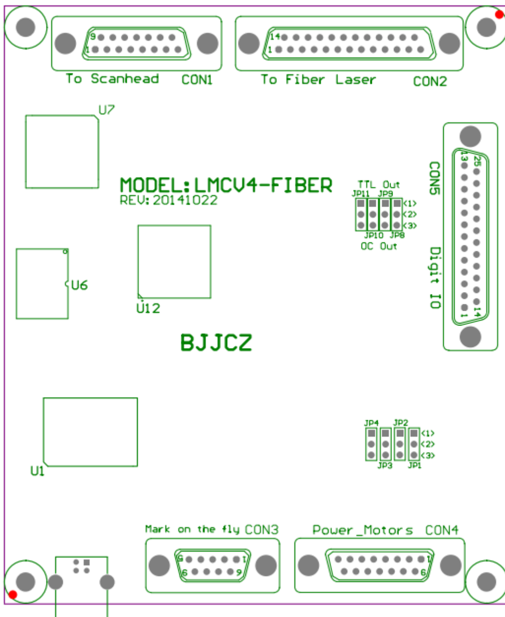
图 1-1 LMC2014 Fiber 控制卡示意图
