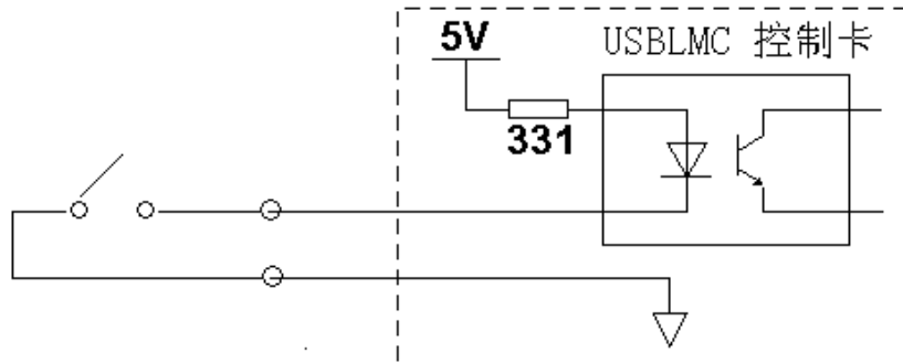
图 2-8 通用输入信号（In4-8/Remark）推荐的连接方案
