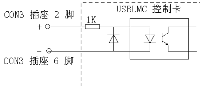
图 2-9 通用输入信号 IN9-13 的接口电路示意图
