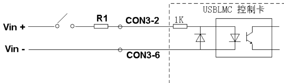
图 2-10 通用输入信号 IN9-13 的推荐的连接方案
