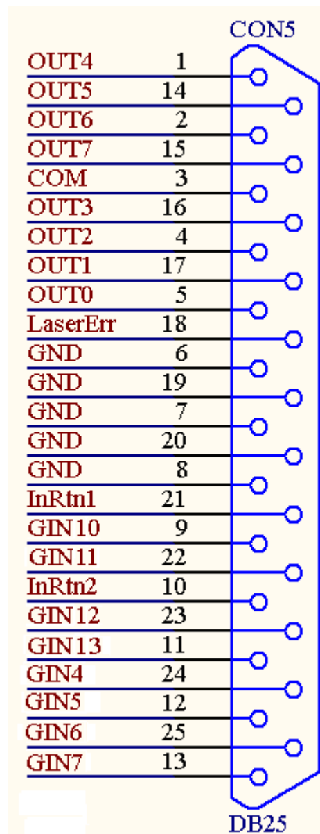
图 2-5 CON5 插座管脚定义示意图
