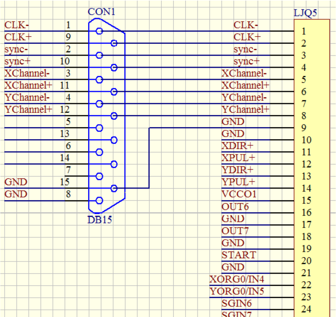
图 2-1 CON1 振镜信号输出示意图
