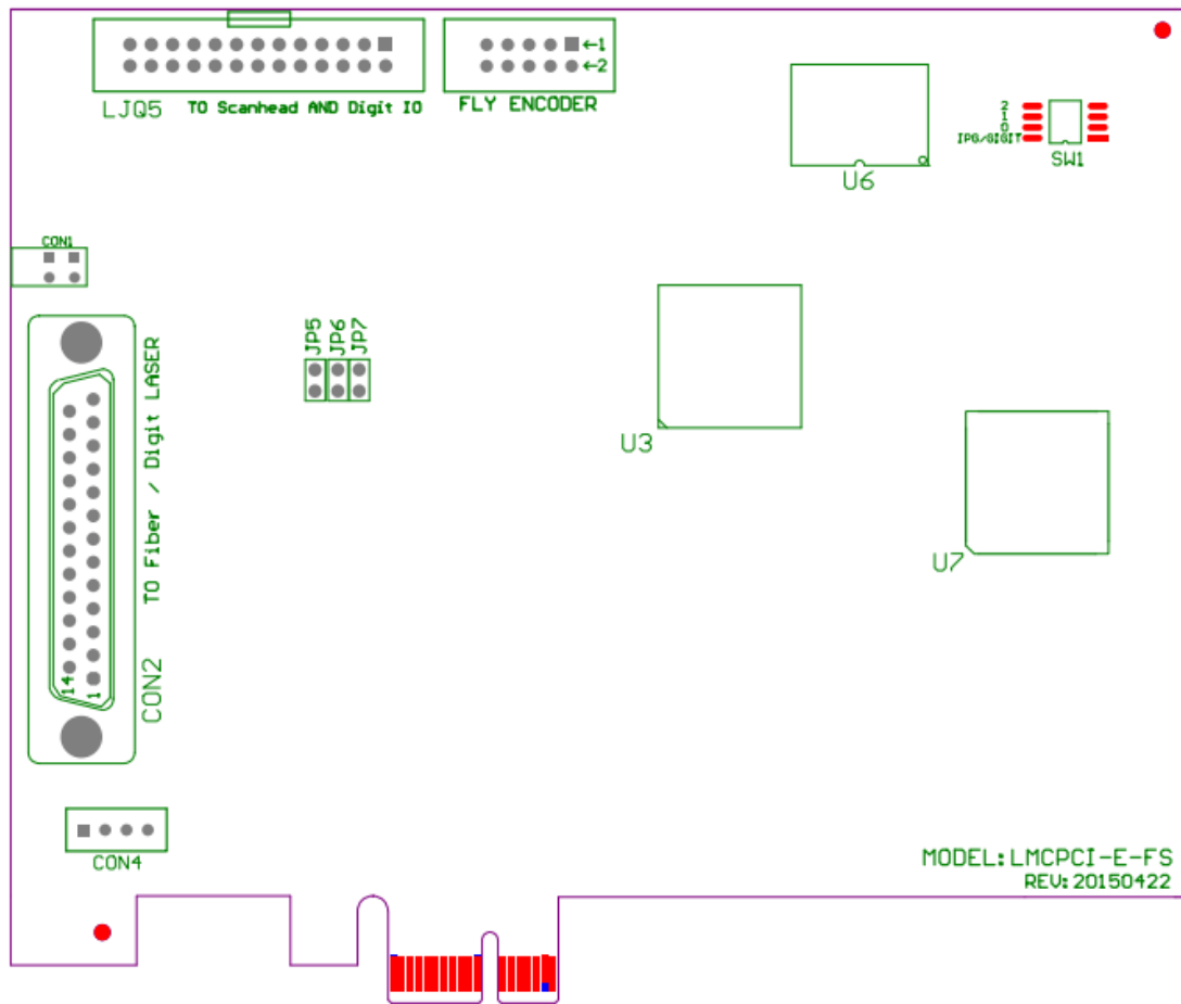
图 2-7 跳线示意图
