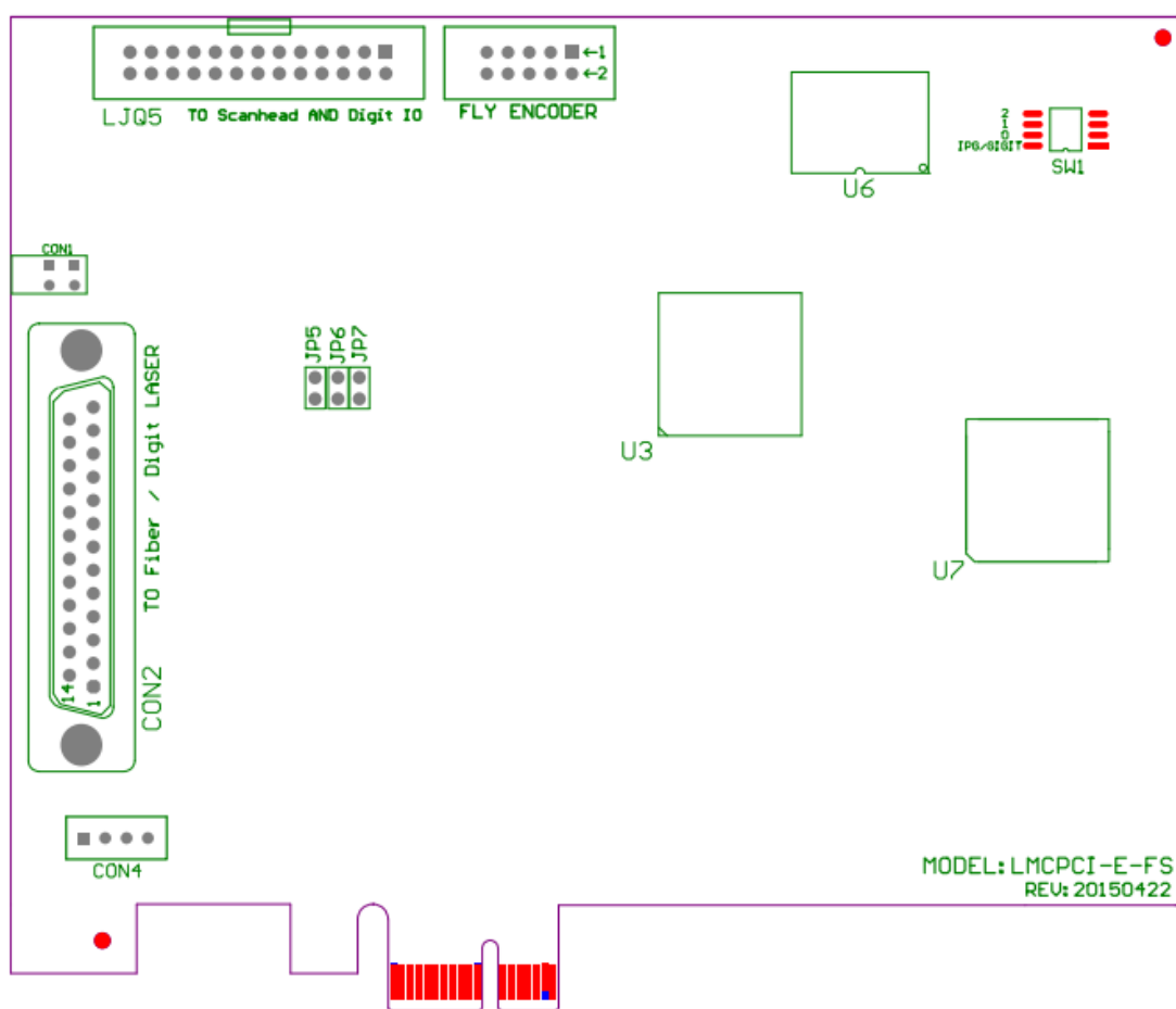
图 1-1 PCIE-FIBER 控制卡外观图
